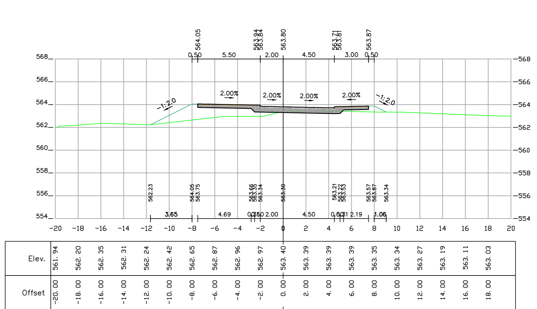
0+180 [Road 1]
