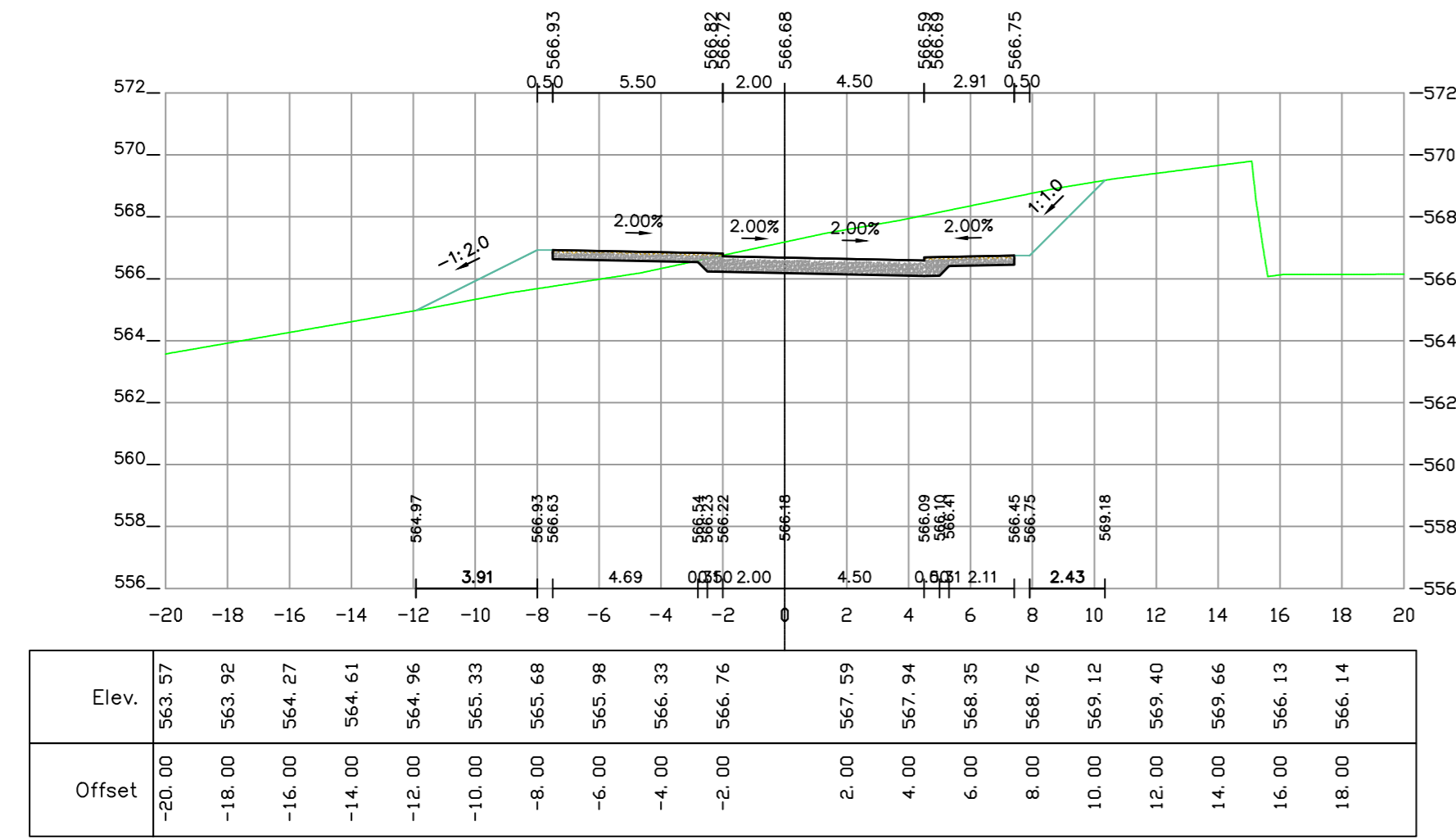
0+080 [Road 1]
